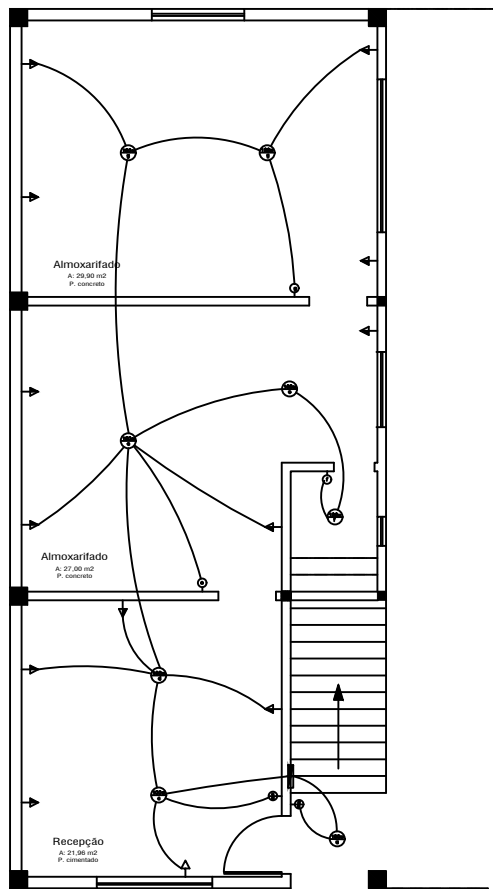
ELÉTRICO TÉRREO A: 98,80 m 2
